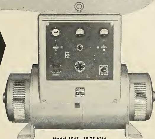
Model 1048—18.75 KVA
