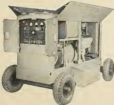
Model 3008-P 37.5 KVA
